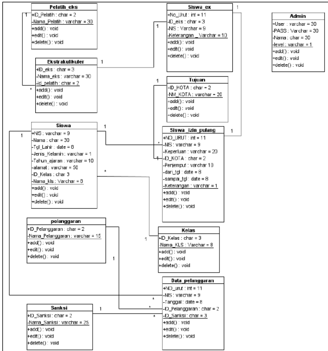
Gambar 3 Class Diagram pada Sistem
